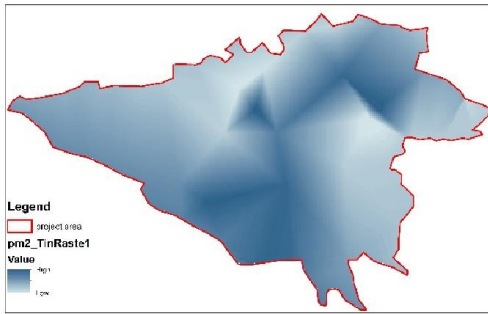
ب: PM_{2.5}
