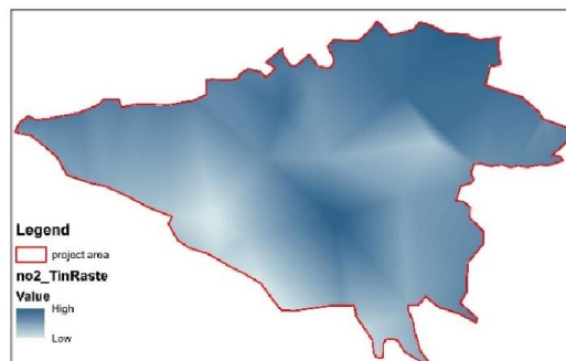
ه: NO_2
