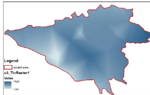
ج: O_3
