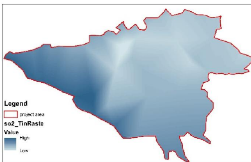
و: SO_2
