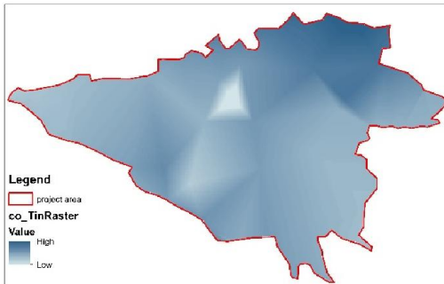
د: CO
