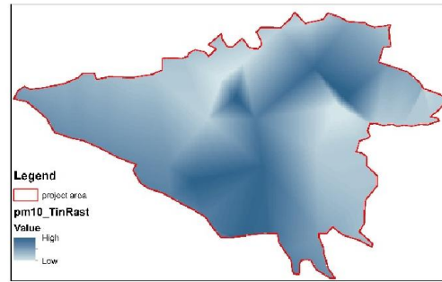
الف: PM_{10}
